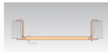
Drzwi rozwieralne bezprzylgowe BF1 (prawe)
