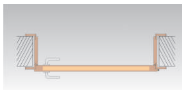
Drzwi rozwieralne przylgowe (prawe)
