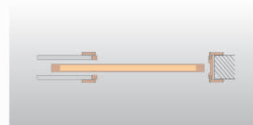
Drzwi przesuwne chowane w kasecie
